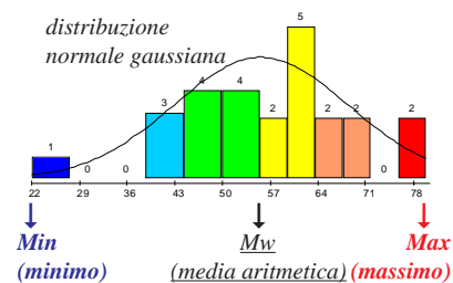
Istogramma della distribuzione di similarità MMinMwMaxX 12-tuplo, secondo IRI_{204,k}
